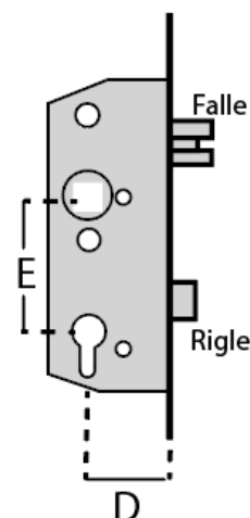
Cylinder: Dråbe
